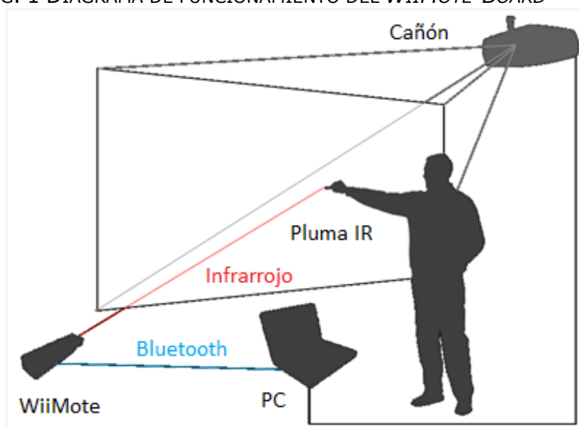
FIG. 1 DIAGRAMA DE FUNCIONAMIENTO DEL WIIMOTE-BOARD
